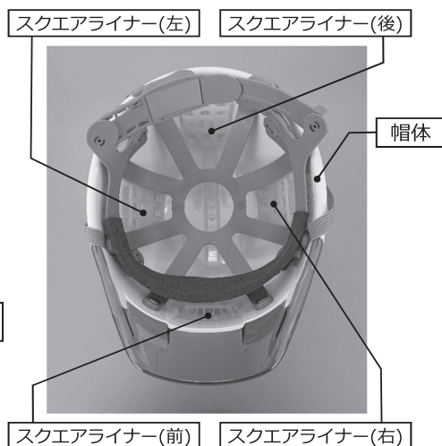
スクエアライナー取付位置
