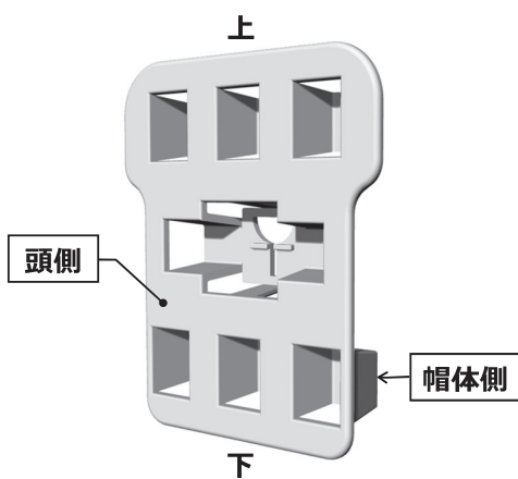
スクエアライナー単品図
